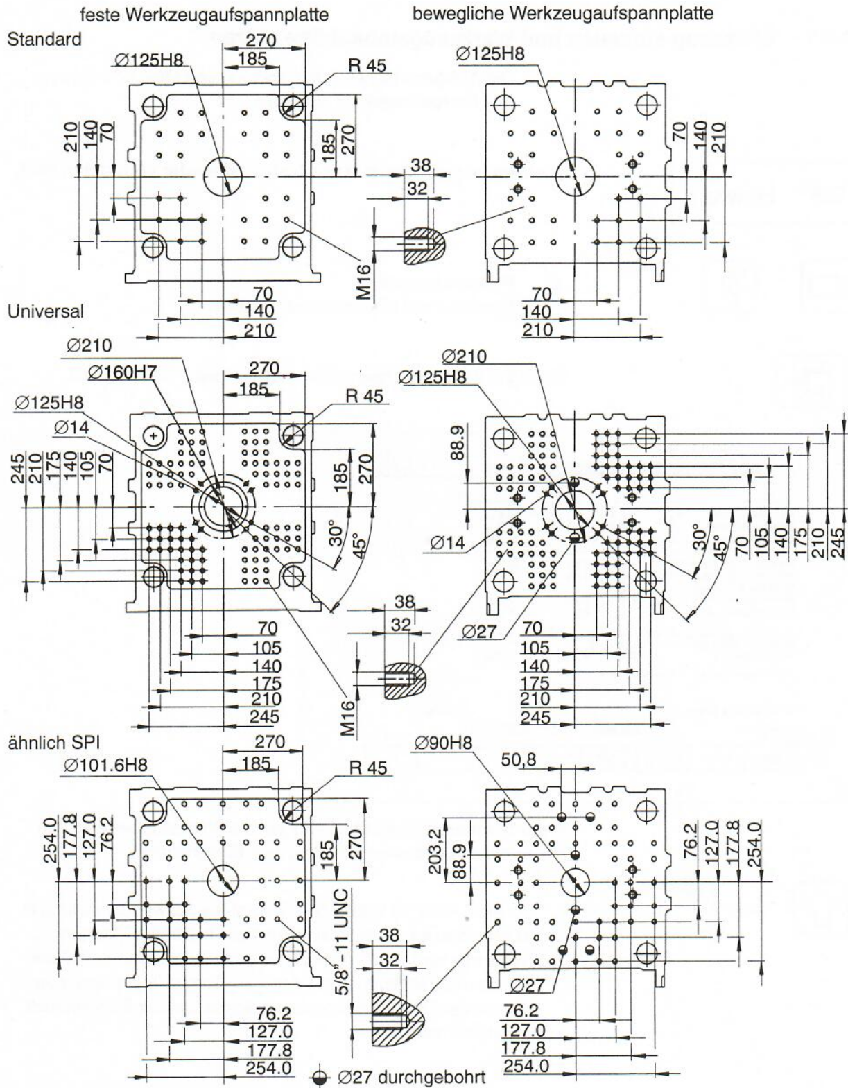
Bild 49: Werkzeugaufspannbohrpläne Ergotech pro 80 / 100
